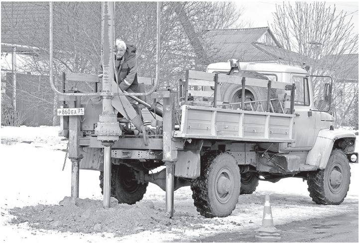
Работает буровая установка в селе Байцуры
